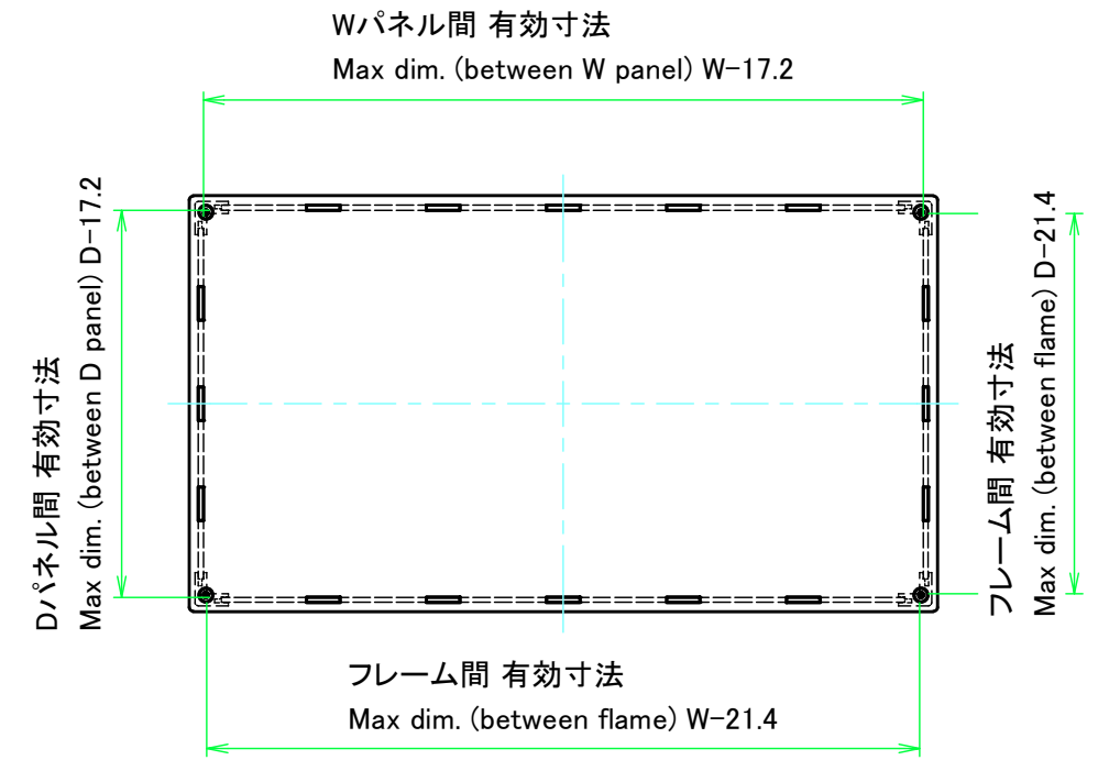
下カバー / Bottom cover
